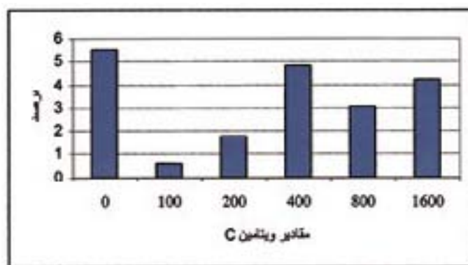
نمودار ۲- میزان تلفات کل دوره در ارتباط با دوزهای مختلف ویتامین C در جیره
